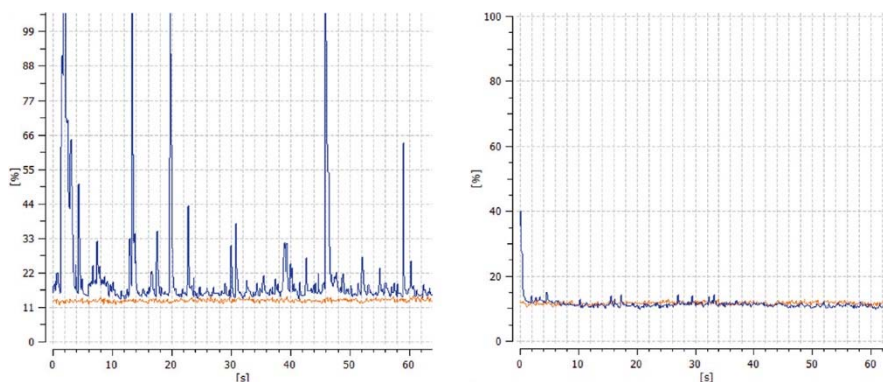
Diagramm für Geräuschklasse >IV (links) bzw. I/1 (rechts)
