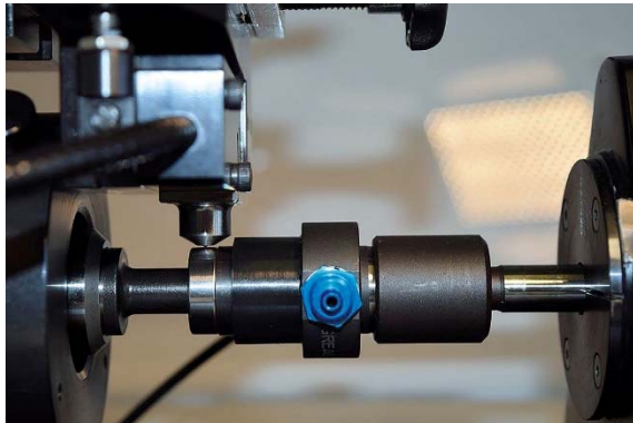
Messaufbau des BeQuiet+
